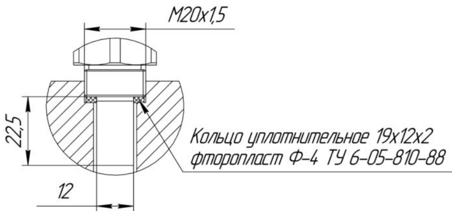
Рис.2. Конструкция фланца для подключения измерительного преобразователя ДТР-3-СМ-М к газовой магистрали.
